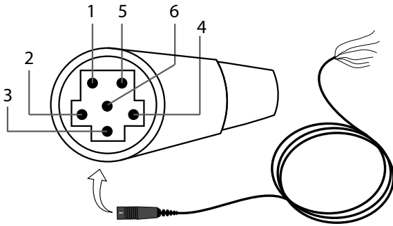
Conector de 6 clavijas de diadema
